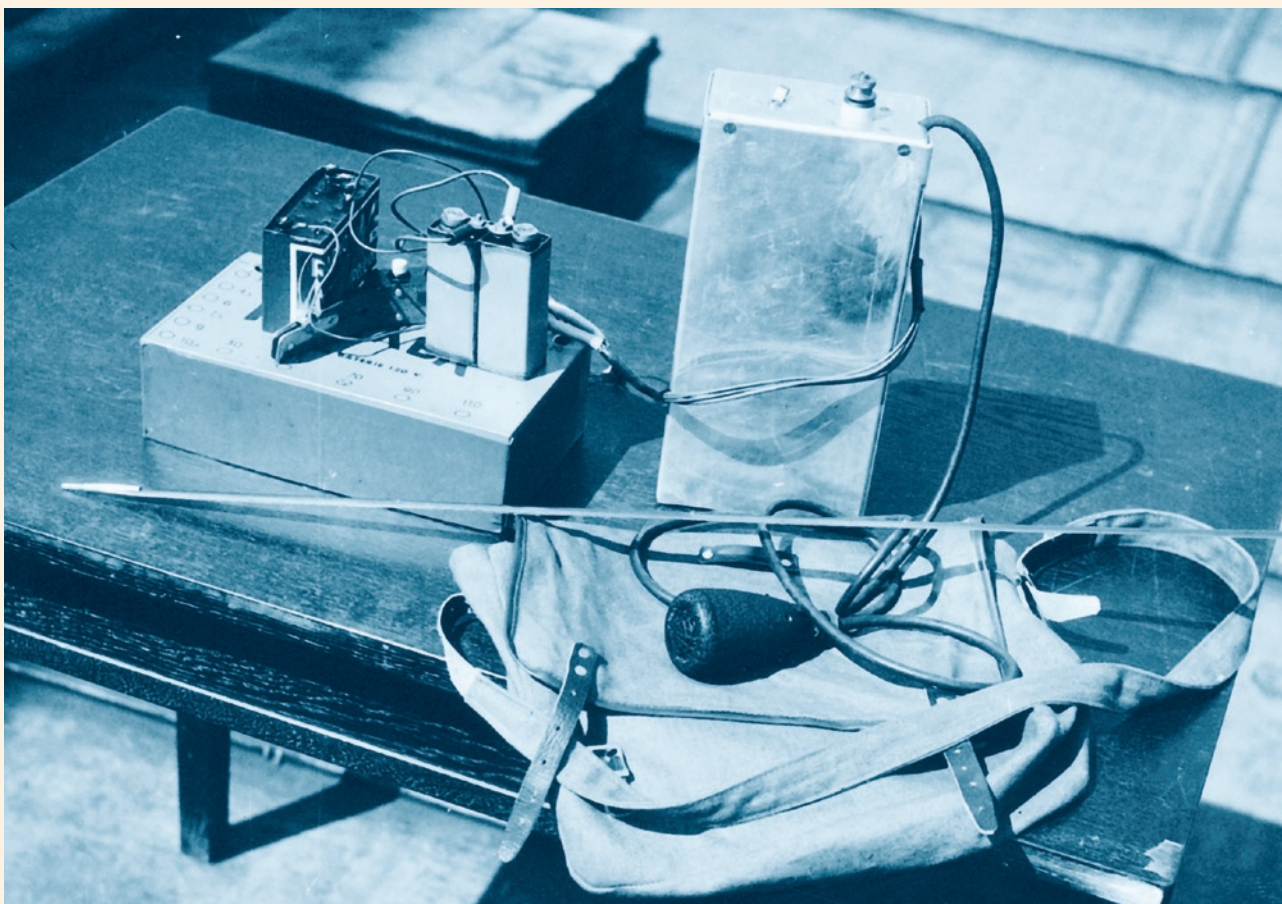
Přenosná krátkovlnná vysílačka (1948)
