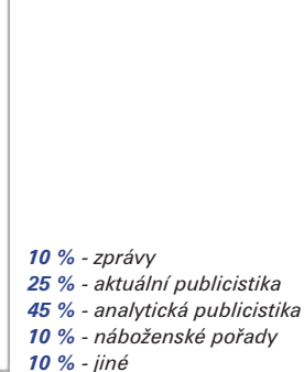
Struktura programu
